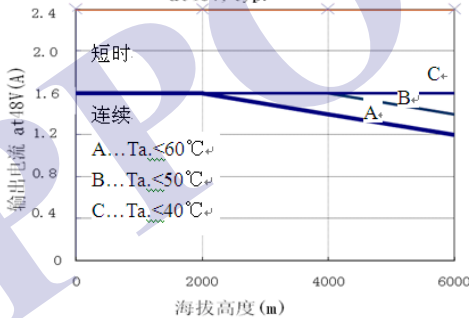
图 6-2-2 输出电流VS海拔高度 at48V, typ.
