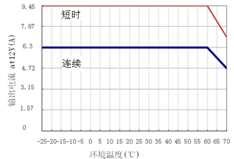
图6-1 输出电流VS环境温度 at 12V, typ.
