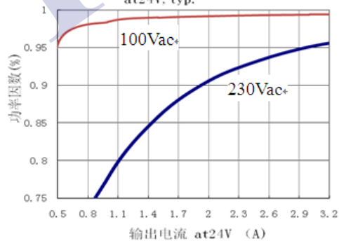
图 1-4-1 功率因数VS输出电流 at 24V, typ.
