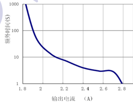
图 3-6-2 额外时间VS输出电流, typ.
