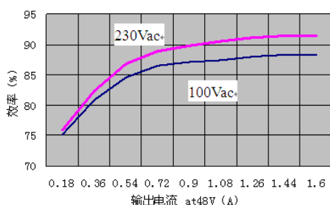
图 1-1-2 效率 VS 输出电流 at 48V, typ
