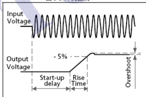
图 3-3 开机曲线
