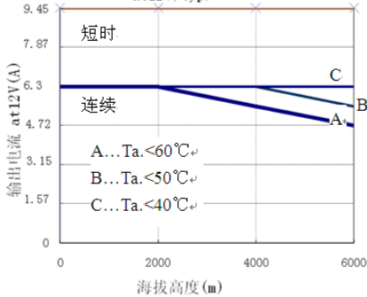
图6-2 输出电流VS海拔高度 at12V, typ.
