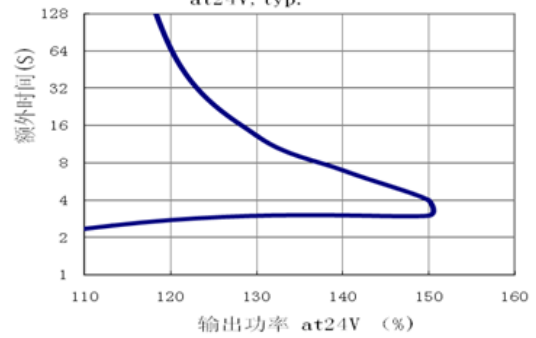
图 3-5-1 额外时间VS输出功率 at 24V, typ.
