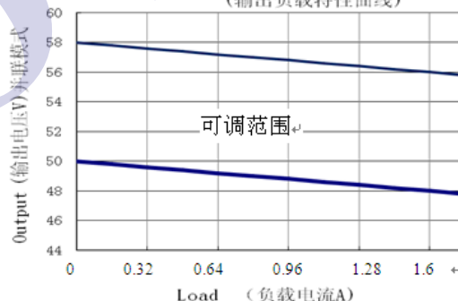
图 3-2-2 Output V-I curve 并联模式 (输出负载特性曲线)
