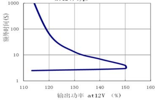
图3-5 额外时间VS输出功率 at 12V, typ.
