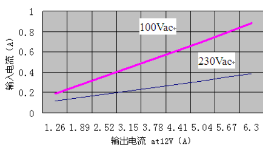
图1-3 输入电流VS输出电流 at 12V, typ
