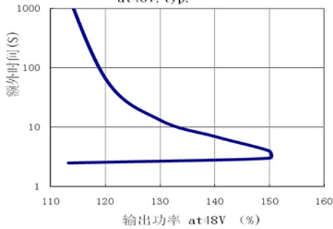
图 3-5-2 额外时间VS输出功率 at 48V, typ.
