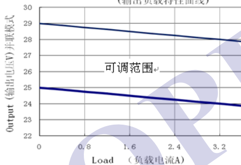
图 3-2-1 Output V-I curve 并联模式 (输出负载特性曲线)
