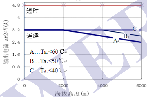
图 6-2-1 输出电流VS海拔高度 at24V, typ.
