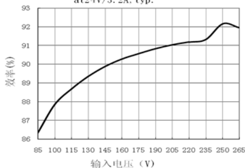
图 1-2-1 效率VS输入电压 at 24V/3.2A, typ.
