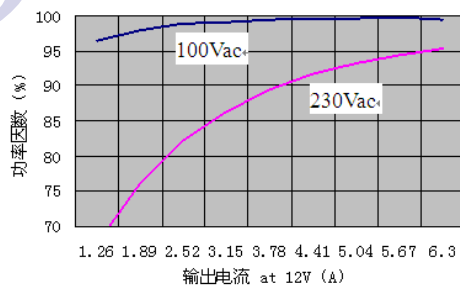
图1-4 功率因数VS输出电流 at 12V, typ
