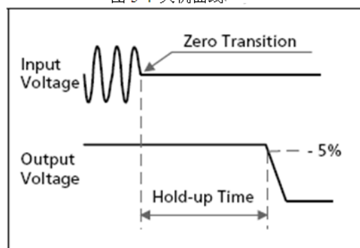
图 3-4 关机曲线
