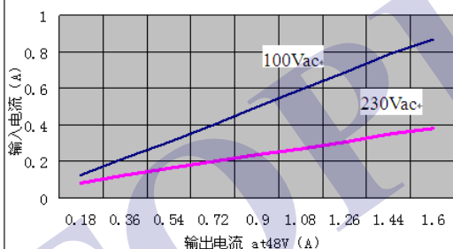
图 1-3-2 输入电流VS输出电流 at 48V, typ
