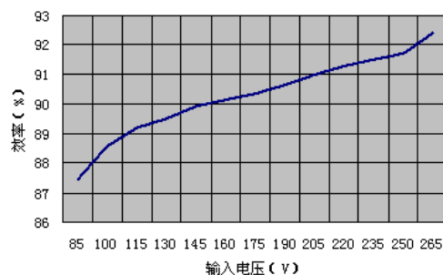
图 1-2-2 效率VS输入电压 at 48V/1.6A, typ
