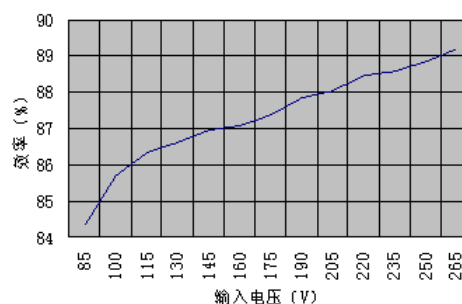
图 1-2 效率 VS 输入电压 at 12V/6.3A, typ
