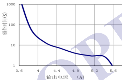
图 3-6-1 额外时间VS输出电流, typ.
