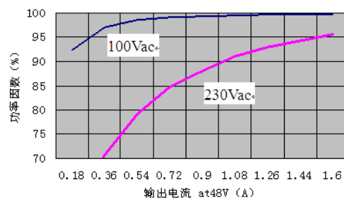
图 1-4-2 功率因数VS输出电流 at 48V, typ
