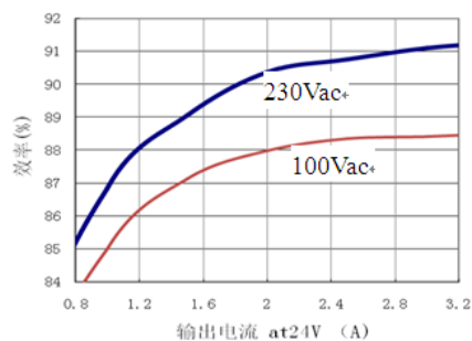
图 1-1-1 效率 VS 输出电流 at 24V, typ.
