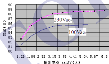
图 1-1 效率 VS 输出电流 at 12V, typ
